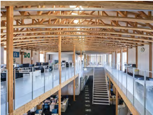
烏森オフィス Kasumori Office Office, 2023
